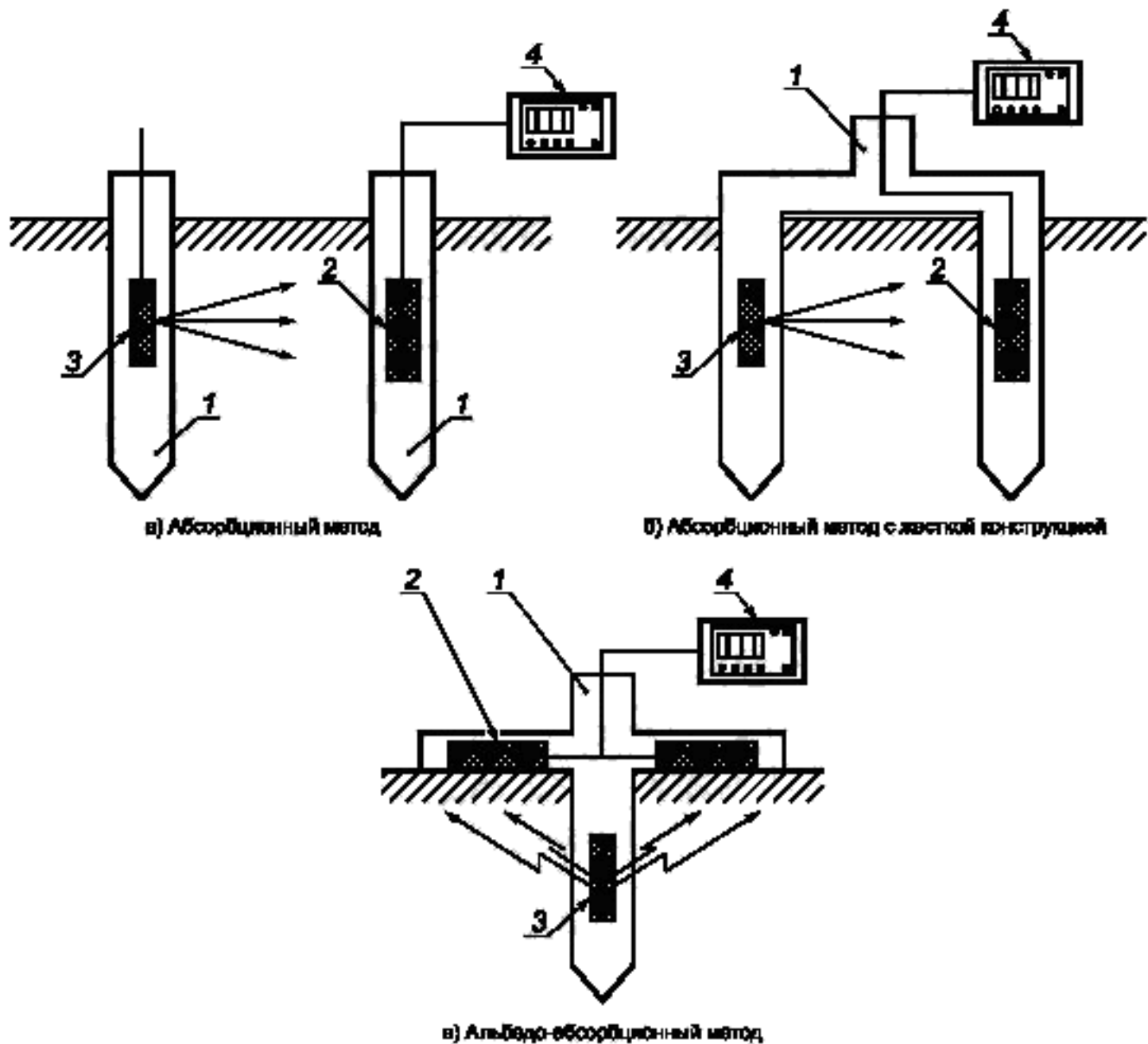
Рисунок 2 — Схемы измерений радиоизотопными плотномерами
