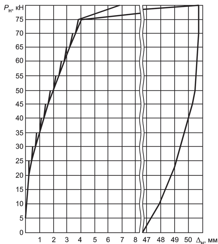
а) График зависимости горизонтального перемещения сваи \Delta_H от нагрузки P_H
