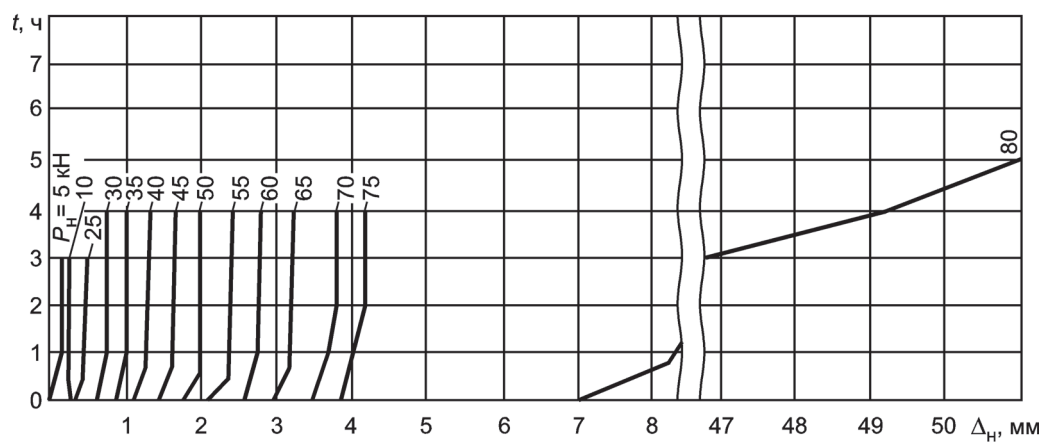
б) График изменения горизонтального перемещения сваи \Delta_H во времени t (по ступеням нагружения)
