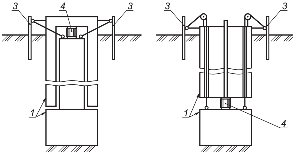
ж) Схемы установок с самоанкерующимися сваями-штампам
